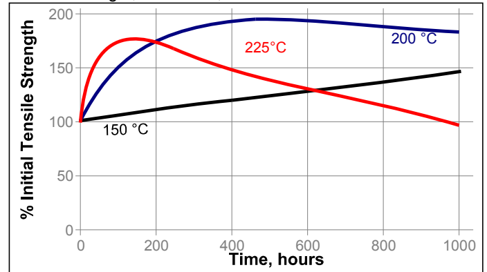
Tensile Strength, ISO 527-3,
